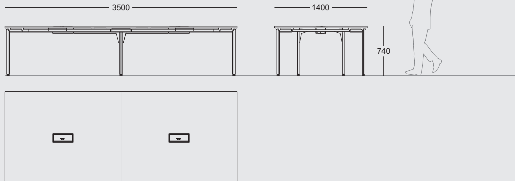
TIPOLOGÍA 3500 x 1400 x h.740 mm
