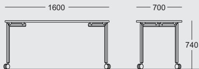
TIPOLOGÍA 1600 x 700 x h.740 mm
