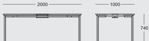
TIPOLOGÍA 2000 x 1000 x h.740 mm
