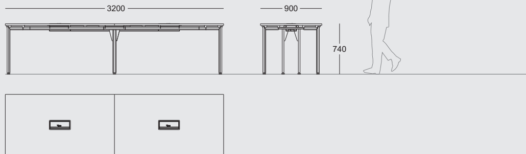
TIPOLOGÍA 3200 x 1200 x h.740 mm
