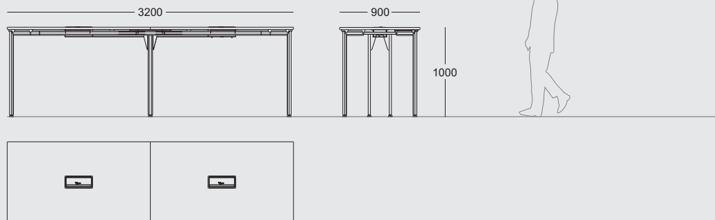
TIPOLOGÍA 3200 x 900 x h.1000 mm
